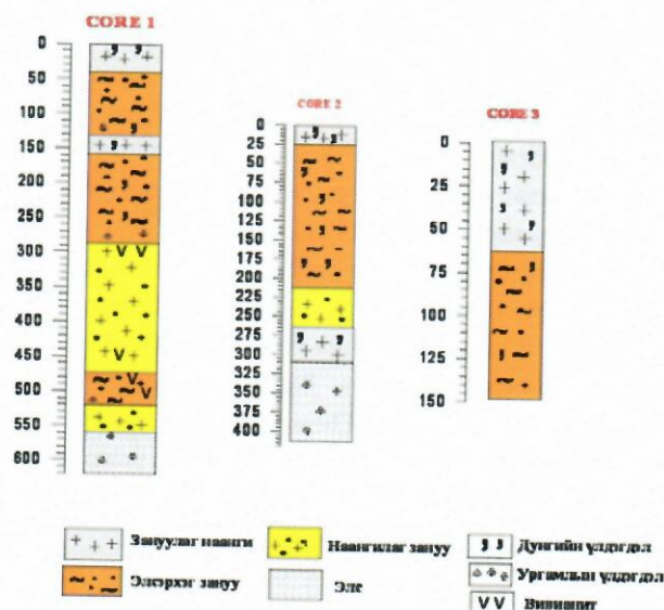
Зураг 2. Доод нуурын хурдасын литологийн тогтоц
