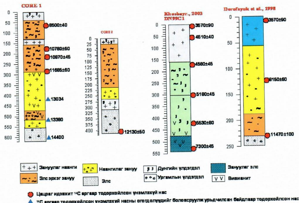
Зураг 3. Доод нуурын хурдсын үнэмлэхүй насны өгөгдөлүүд
