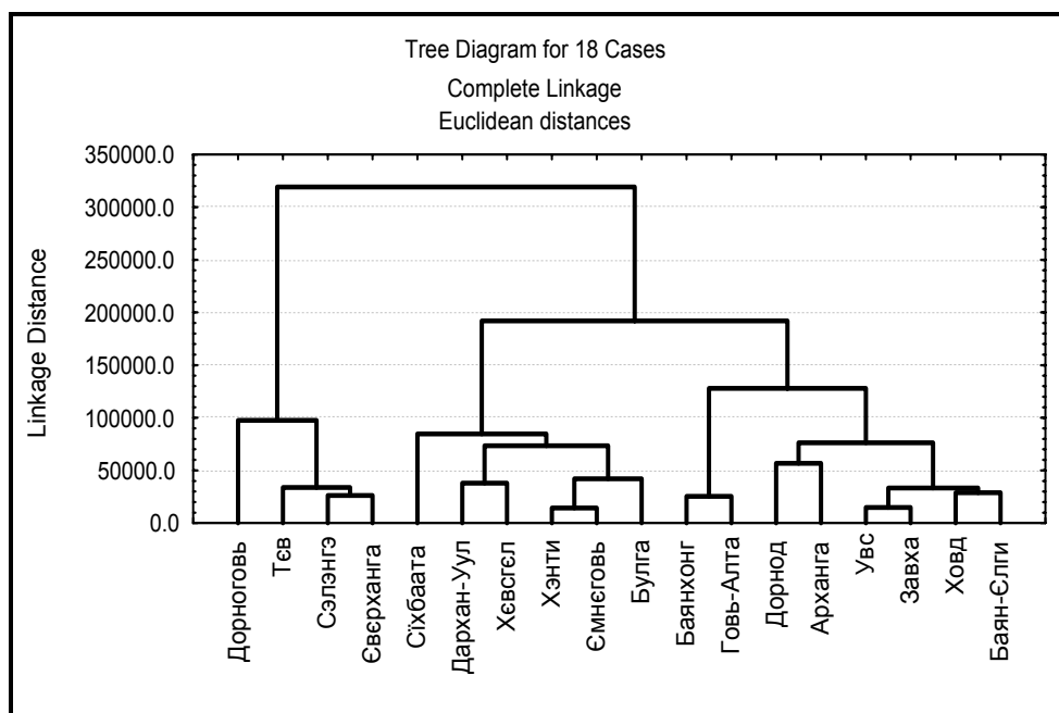
Зураг 7. Дендрограмм
