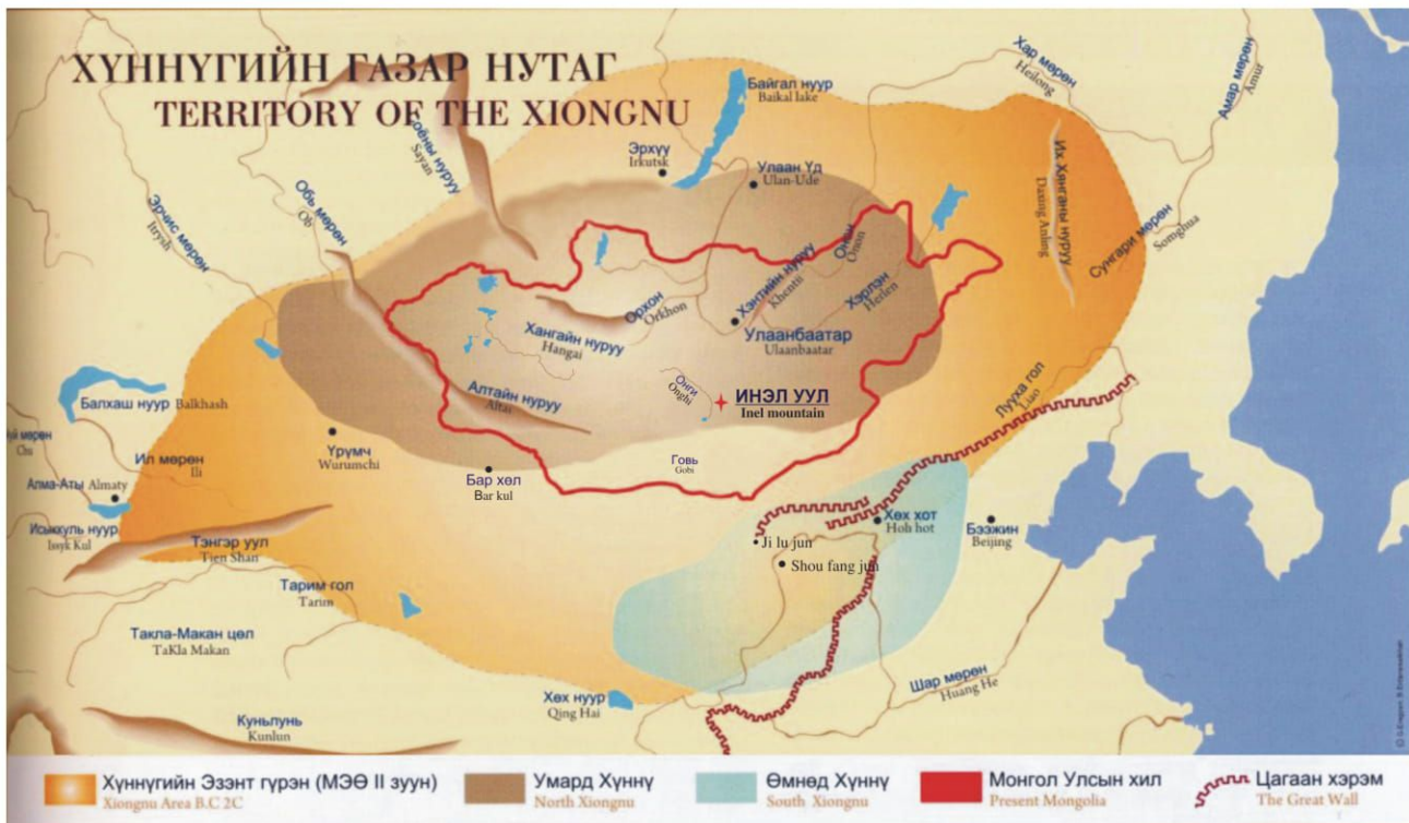
Зураг 1. Хүннүгийн газар нутаг дахь Инэл уулын байршил (МЭӨ II-МЭ I зуун)
