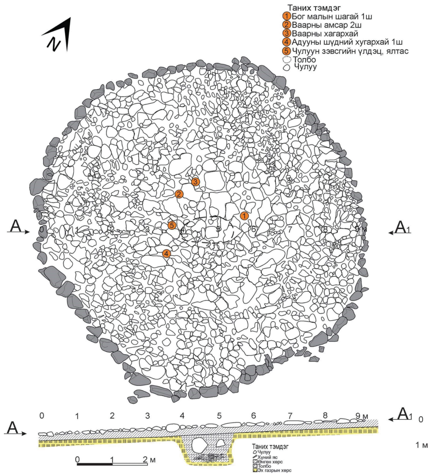
Зураг 3. Харуулын гозгор уулын бушины гар зураг
